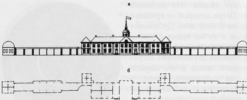
Дворец в Дальних Дубках. Фиксационный чертеж и план. 1748 г.
