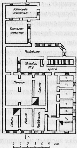
План нижнего этажа 1911 г.
