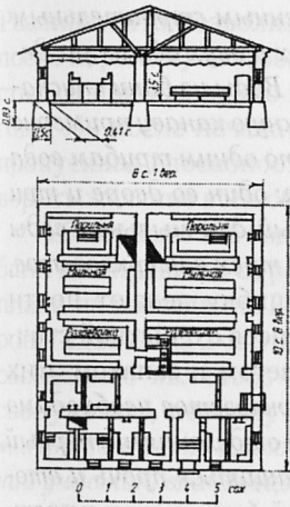
Проект Городской бани на 40 человек Уставом Губернии Самбоксского в с. Самарском 1898 г. Составил Военный инженер подполковник Вереженин
