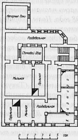
План Верхнего этажа 1911 г.
