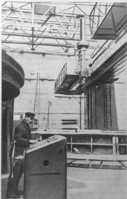
Выполнение заказа «Большой Волги» на крупнейшем в СССР карусельном станке Металлического завода. 1939 г. Фотография.
