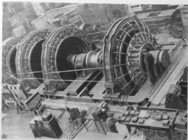
Электрооборудование слябинга для Запорожстали, впервые изготовленное на «Электросилев». Май 1936 г. Фотография.
