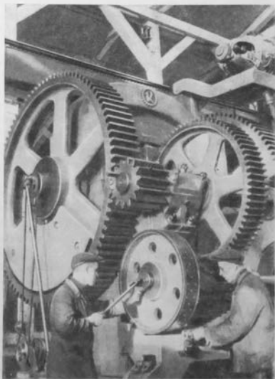
Испытание 700-тонного пресса, изготовленного ленинградцами для Горьковского автозавода. Январь 1937 г. Фотография.
