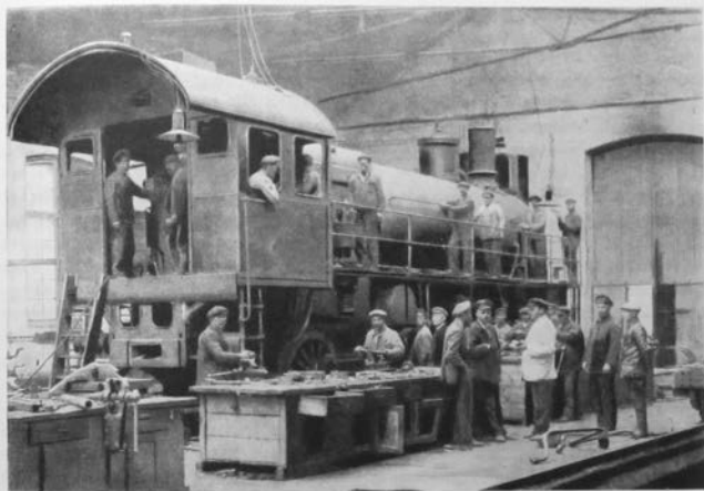
Восстановление паровозов на Невском машиностроительном заводе. 1925 г. Фотография.
