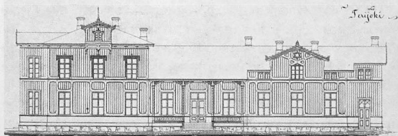
Фрагмент проекта железнодорожного вокзала Терийоки, чертеж 1871 г. Национальный архив Финляндии
